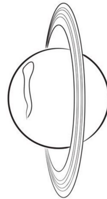
Uranus
