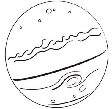
Jupiter
