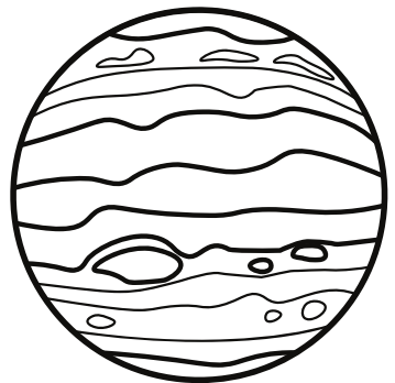
Jupiter
